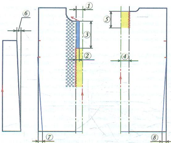
Схема моделювання елементів традиційного крою «в перекидку» для чоловічої сорочки. Зліва направо: бічний клин, половина крою пілочки, половина крою спинки
