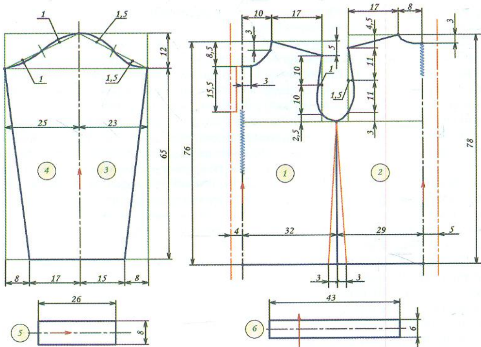
Схема сучасного крою чоловічої сорочки із моделюванням під вишиванку на середній зріст із обхватом грудей 100 см. Деталі крою (на схемі позначено цифрами в кружечках): 1 — пілочка, 1 деталь; 2 — спинка, 1 деталь; (3—4) — рукав, 2 деталі; 5 — манжета, 2 деталі; 6 — комір, 1 деталь. *3 — передня частина рукава, 4 — його задня частина
